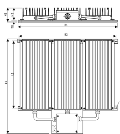
Maßbild, Bauform 2
