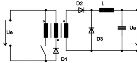
Schaltprinzip Durchflusswandler
