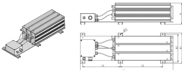
Maßbild, Bauform 3
