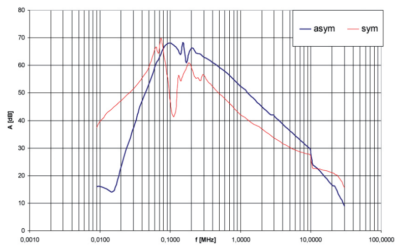
Dämpfungsverlauf CNW107.3
