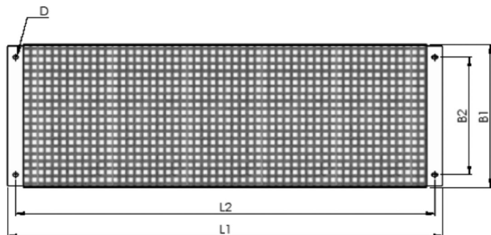
Maßzeichnung Berührungsschutz / Abdeckung
