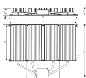
Maßbild, Bauform 3
