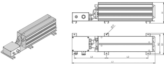
Maßbild, Bauform 2
