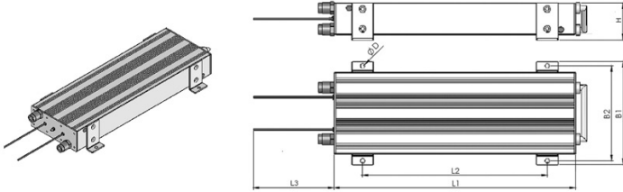
Maßbild, Bauform 1
