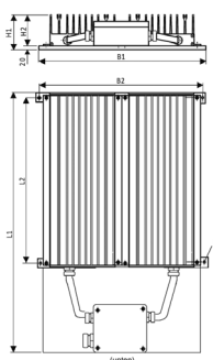
Maßbild, Bauform 1
