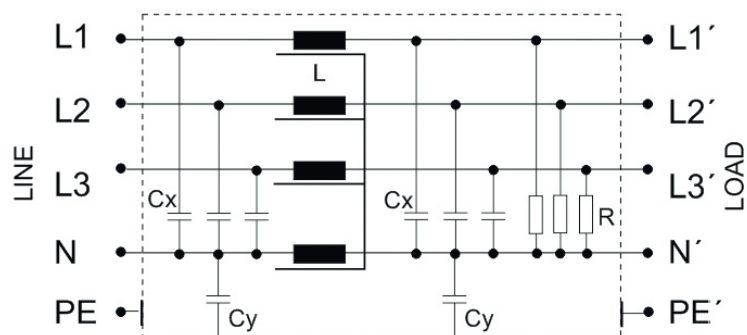
Schaltungsbeispiel
