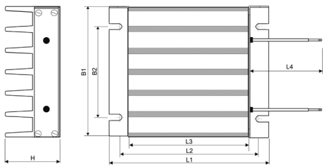
Bauform IP65 / TS
