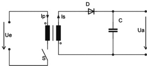
Schaltprinzip Sperrwandler
