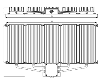
Maßbild, Bauform 4
