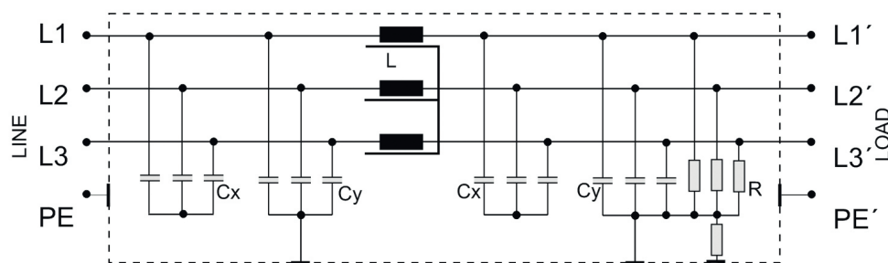
Schaltungsbeispiel
