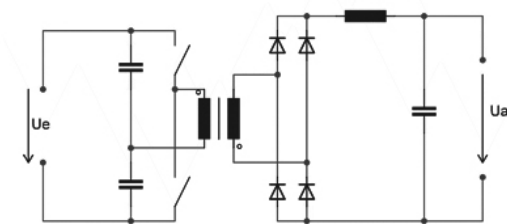
Schaltprinzip Halbbrücken-Gegentaktwandler
