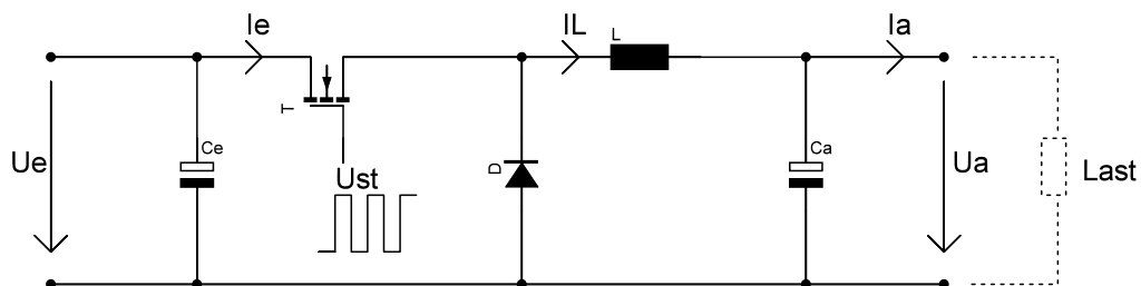
Schaltungsprinzip Tiefsetzstellerdrossel
